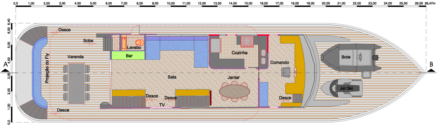
PLANTA LAYOUT 2º PAVIMENTO ESCALA 1:75
