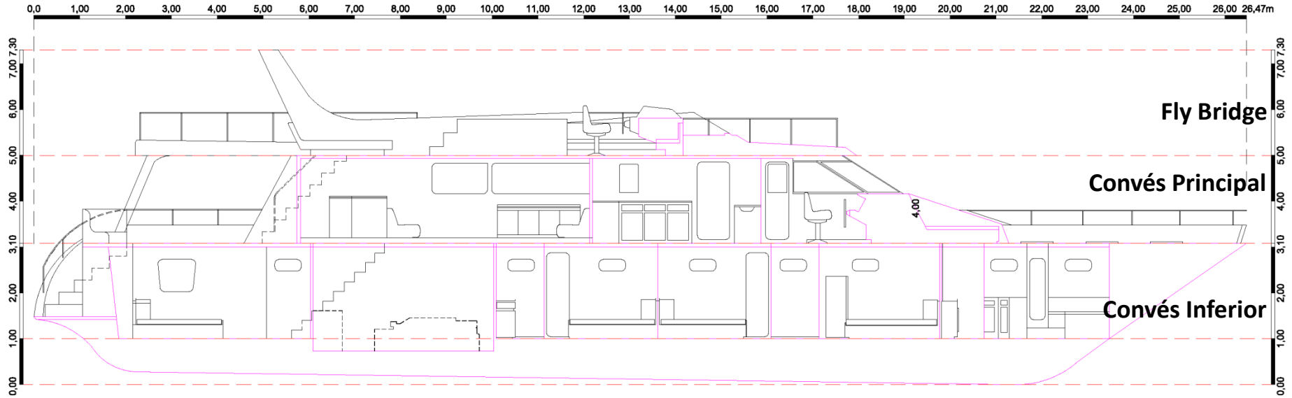
CORTE A-B ESCALA 1:75
