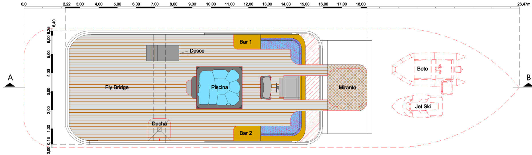
PLANTA LAYOUT FLY ESCALA 1:75
